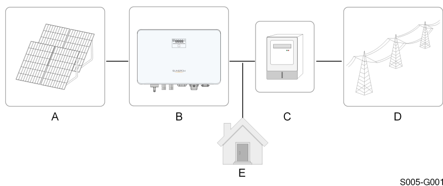
figure 2-1 Application de l'onduleur dans un système d'alimentation photovoltaïque
