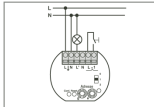
Aansturing via: impulsgever schakelaar wisselschakelaar
