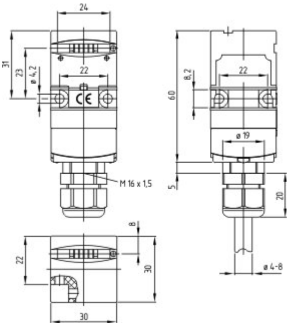
Maatschets (basistoestel)
