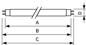
TL-D De Luxe 36W/965
