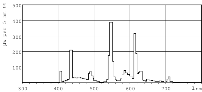
Lichtkleur /840
