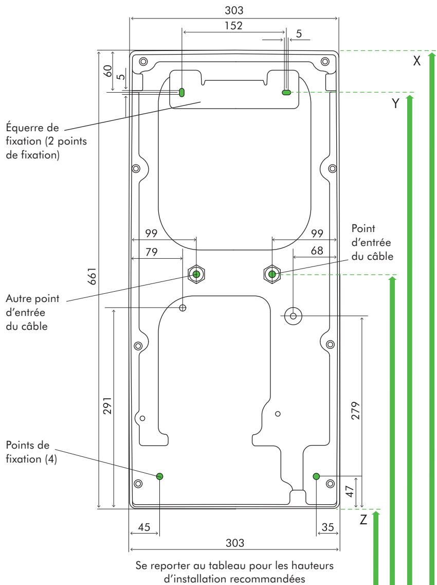
SCHÉMA DU DOS DE L'APPAREIL
