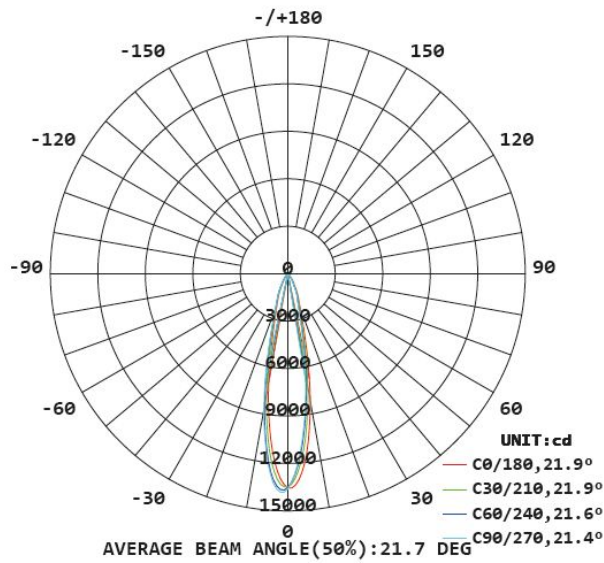
Lumen diagramme de distribution
