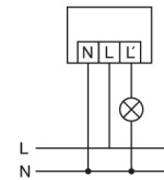
Standardbetrieb mit zusätzlichem Anschluss von externen Lasten
