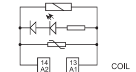
Exemple: AC
