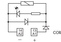
Exemple: DC
