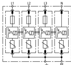
Schéma de principe du circuit DG M TNS CI 275
