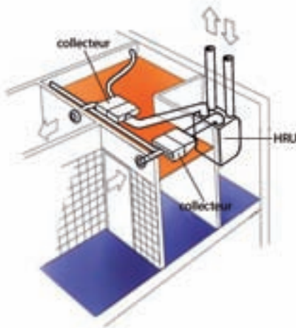
1. Montage des collecteurs d'air en faux-plafond.
