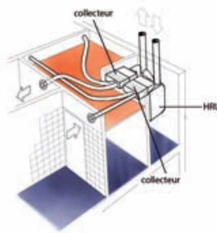
2. Montage des collecteurs dans la même pièce que le HRU.
