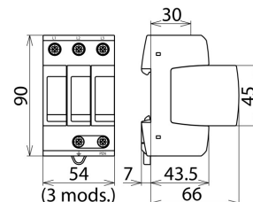
Dimensions DG M TNC 275
