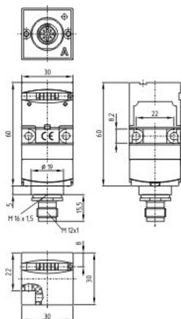
Plan dencombrement (composant de base)
