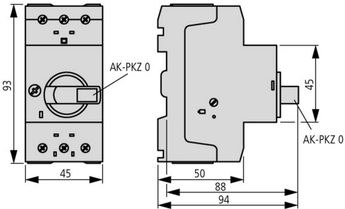
Disjoncteurs-moteurs avec manette rotative cadenassable PKZM0-...+AK-PKZ0
