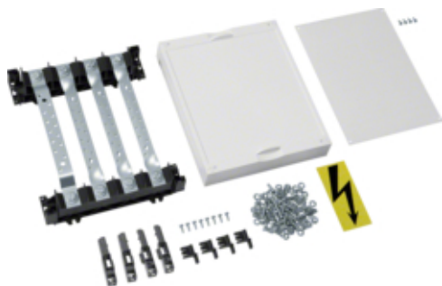
Unité équipement avec jeu de barres tétra Univers cu 25x4mm 250A 1 travée h300mm
