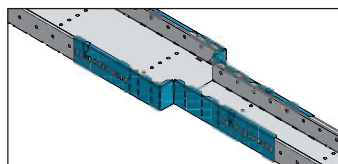
Asymmetrisch reduceren met koppel/reduceerstuk 896.00.00 en koppelplaat 801.00
