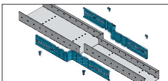
Symmetrisch reduceren met 2 stuks koppel/reduceerstuk 894.00.00
