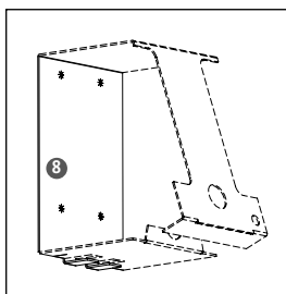
Gabarit de perçage Close-up®
