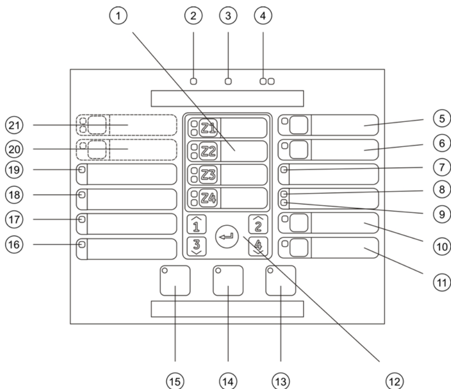
Figure 8 : Interface utilisateur pour les centrales de détection incendie à deux et quatre zones
