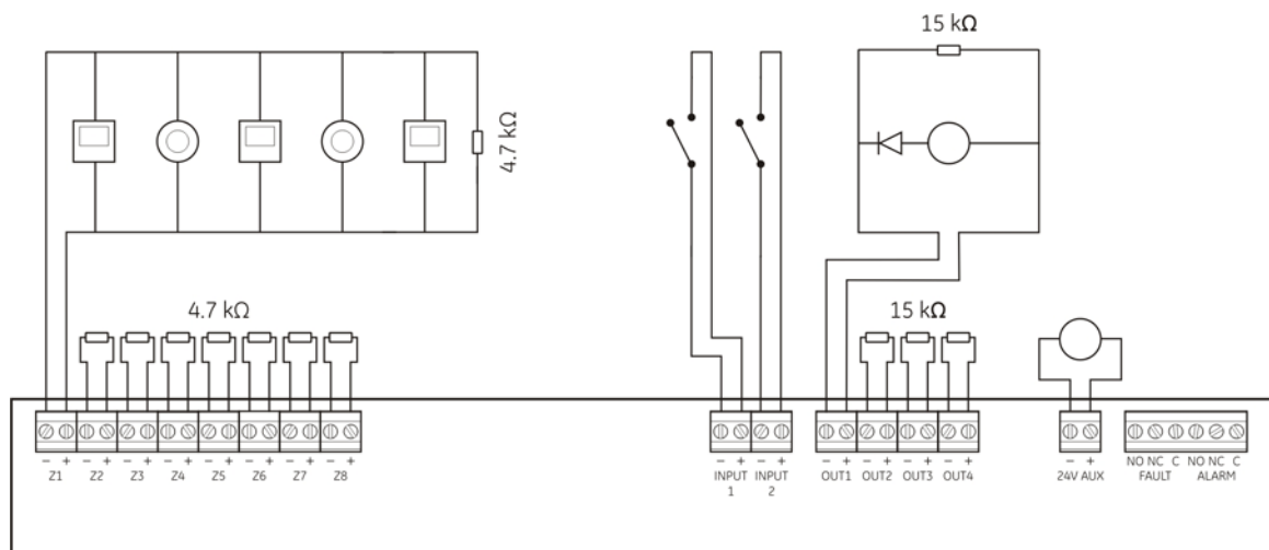
Figure 4 : Présentation des raccordements de la centrale de détection
