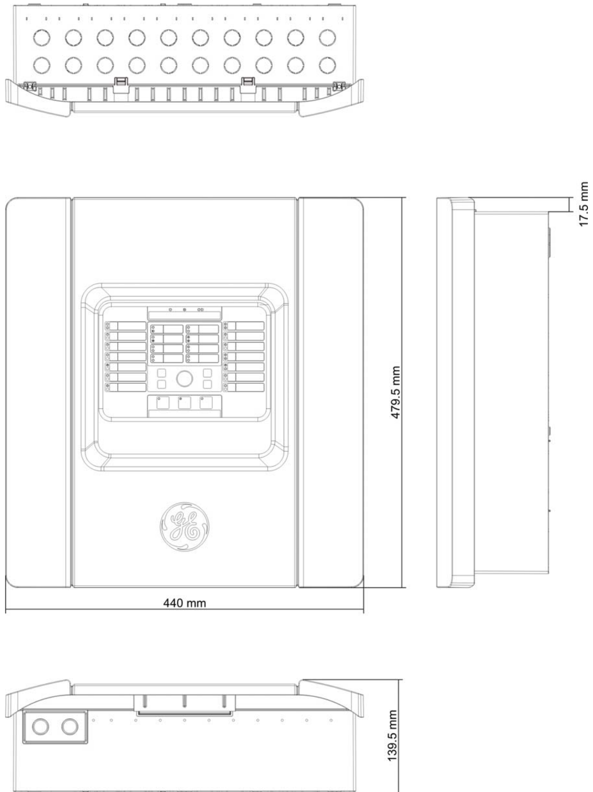
Figure 15 : Armoire à huit zones avec couvercle
