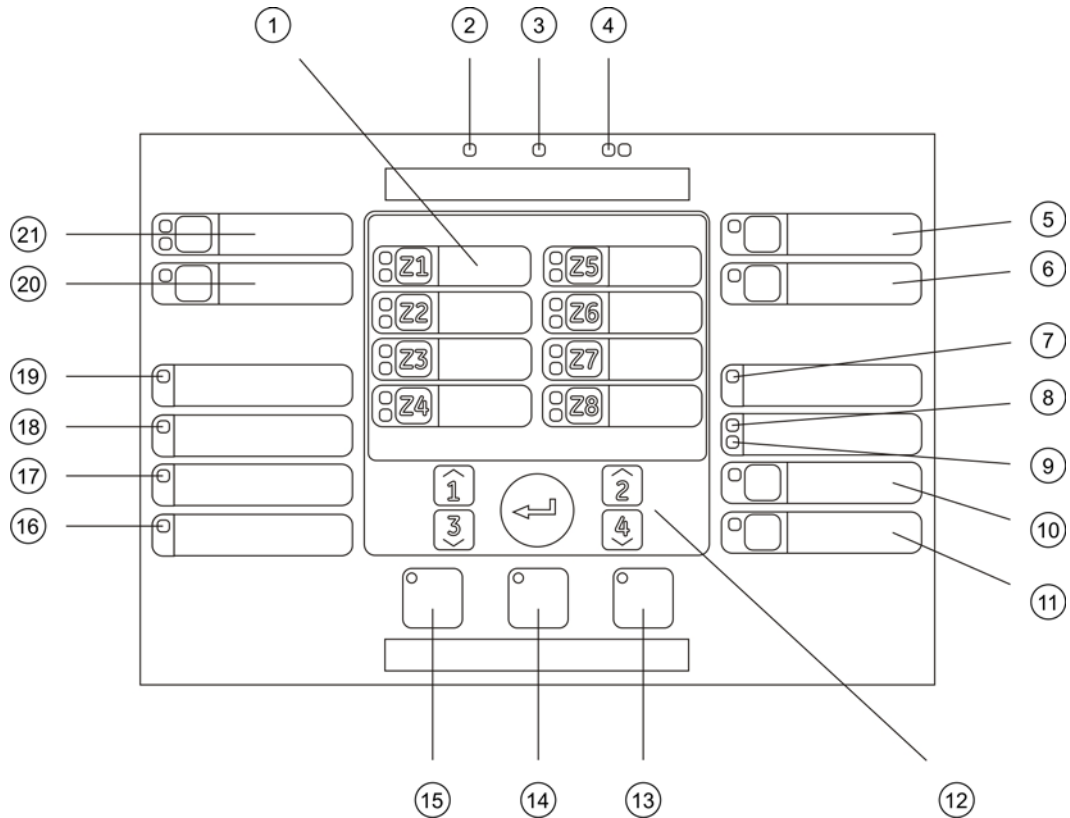
Figure 9 : Interface utilisateur pour les centrales de détection incendie à huit zones
