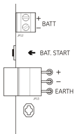
Figure 12 : Bouton de mise en route de la batterie
