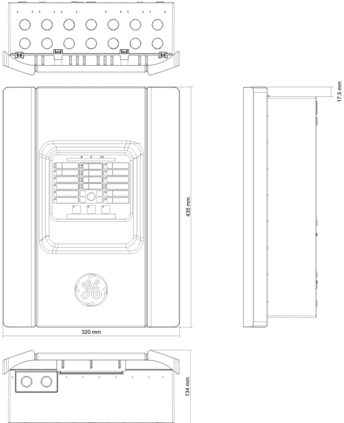
Figure 13 : Armoire à deux et quatre zones avec couvercle
