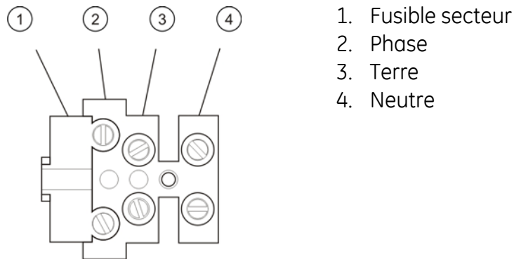
Figure 5 : Raccordement de l'alimentation secteur
