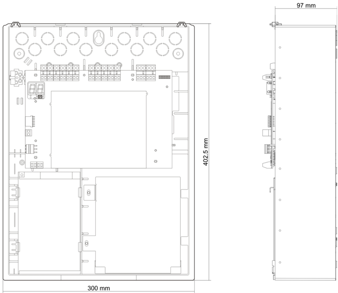
Figure 14 : Armoire à deux et quatre zones sans couvercle
