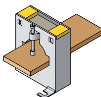
TC à barre ou câble passant
