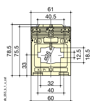
TCB 44-63 et T2CB 44-63
